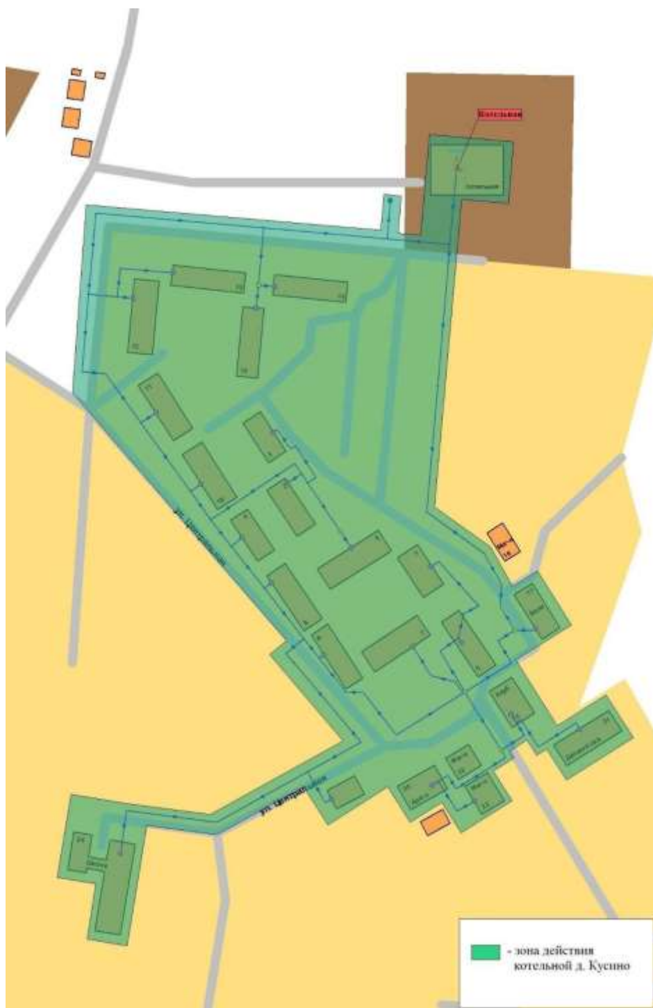
Рисунок 7 - Зона действия котельной МП «Жилищное хозяйство»
