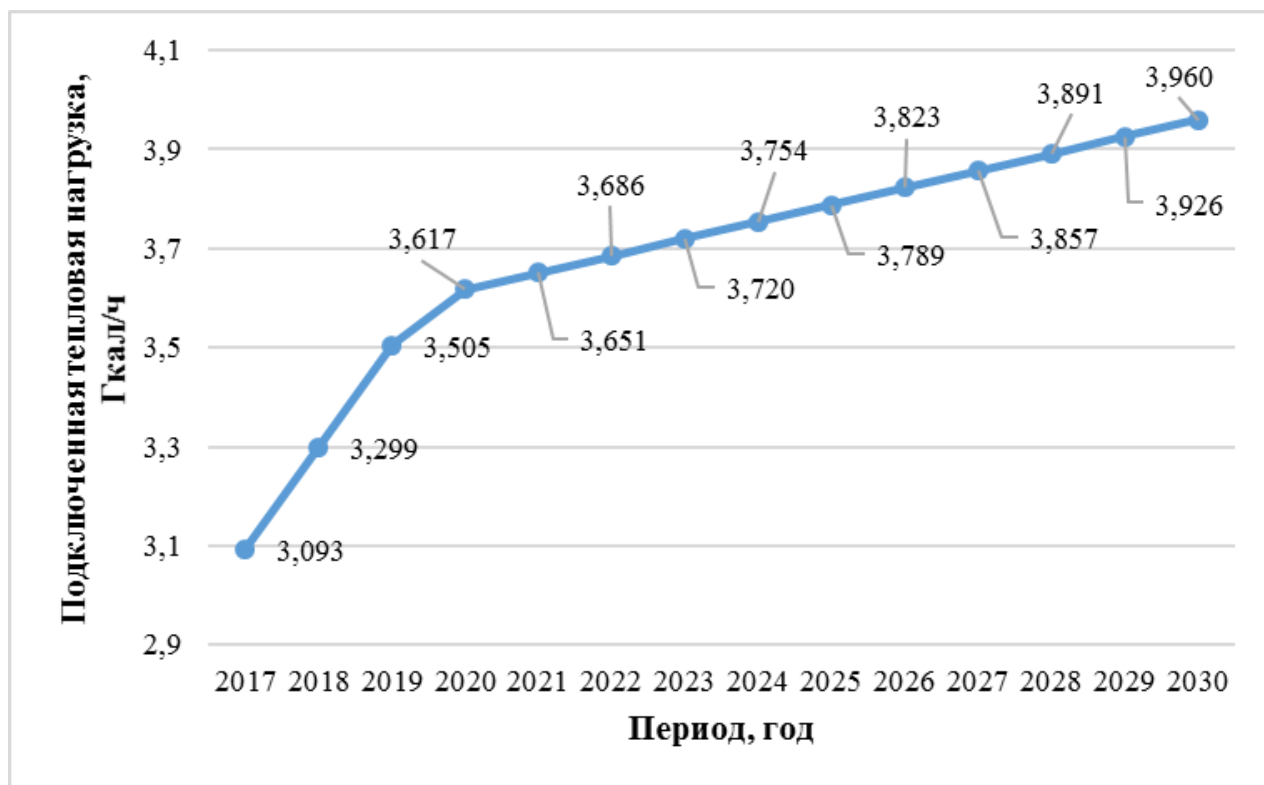
Рисунок 14. Изменение тепловой нагрузки
