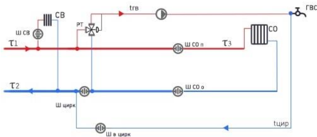
Рисунок 9. Схемы присоединения потребителей
