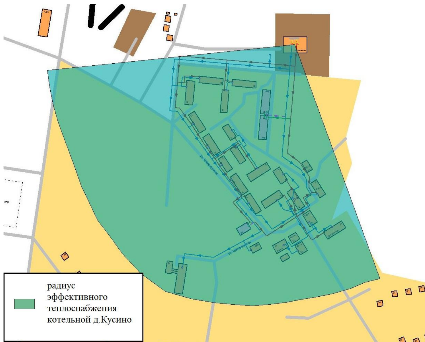
Рисунок 18. Радиус эффективного теплоснабжения от котельной
