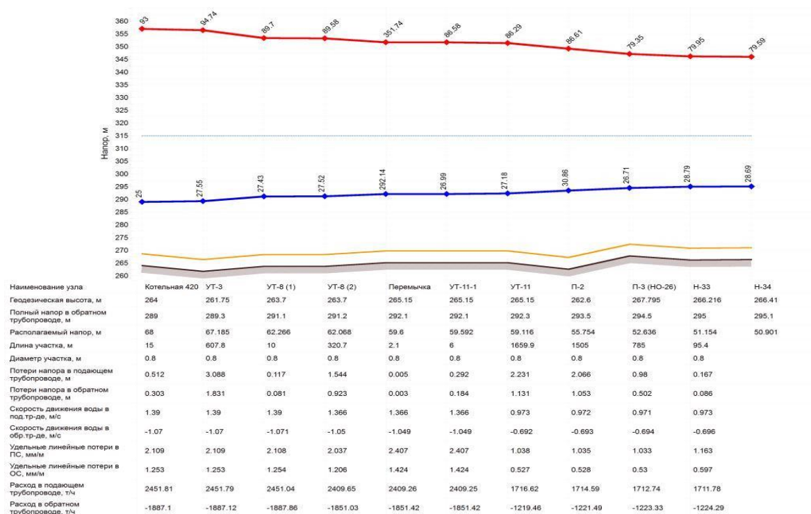
Рисунок 16. Пьезометрический график
