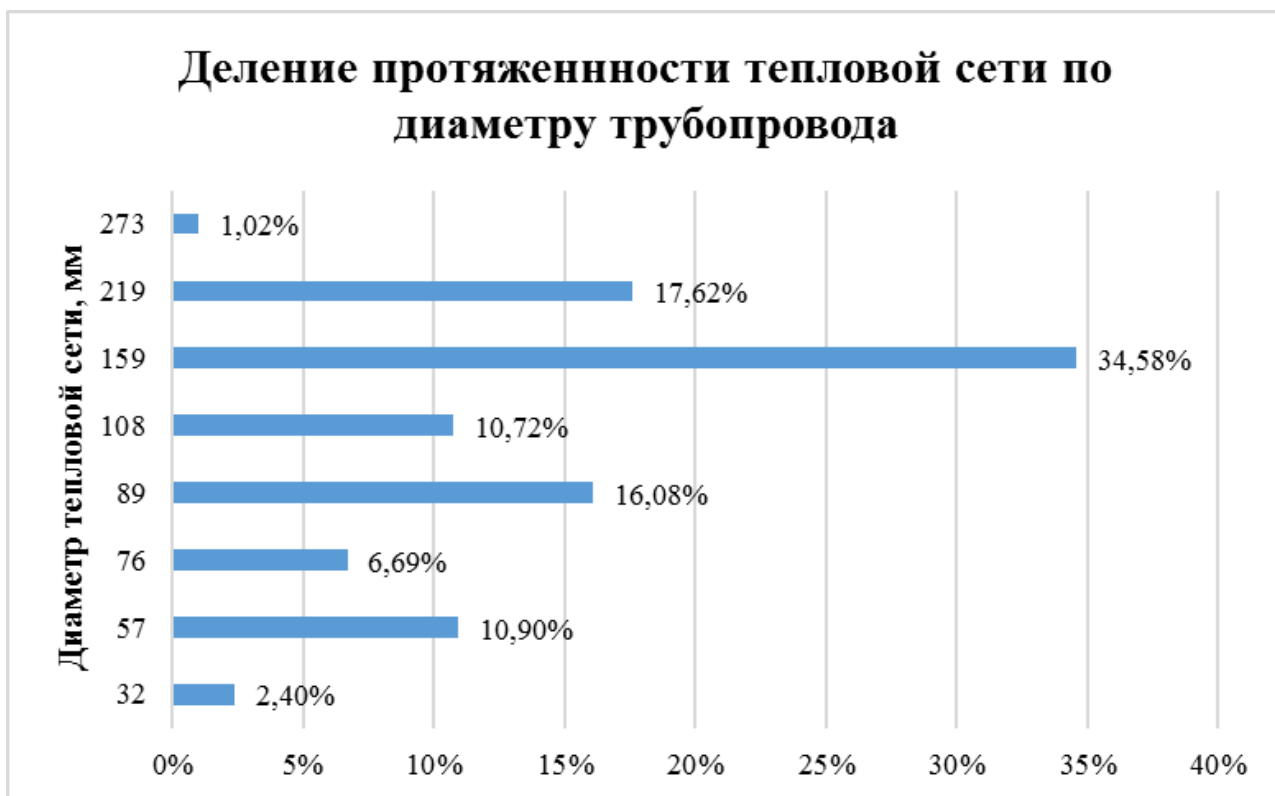
Рисунок 6. Деление протяженности тепловой сети по диаметру трубопроводов
