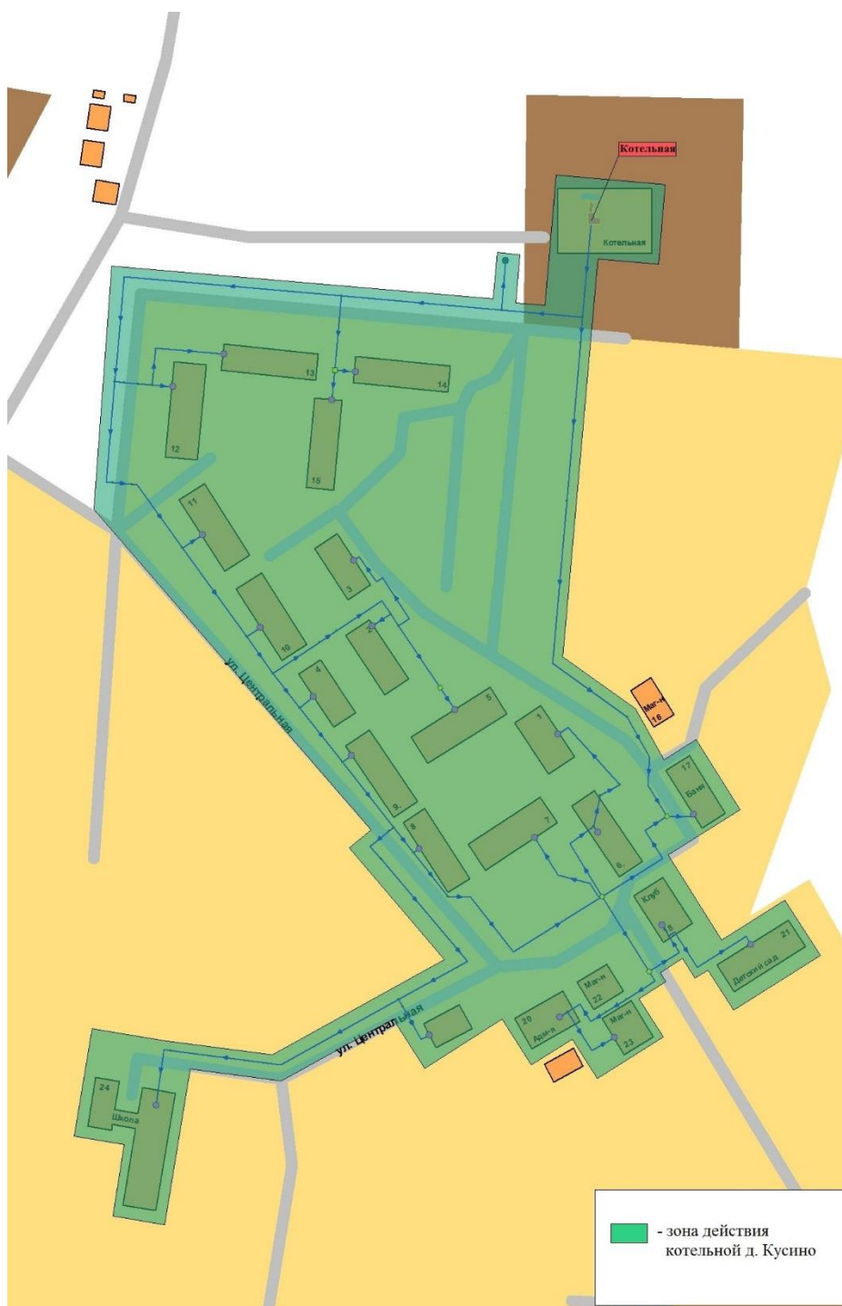
Рисунок 10. Зона действия котельной МП «Жилищное хозяйство»
